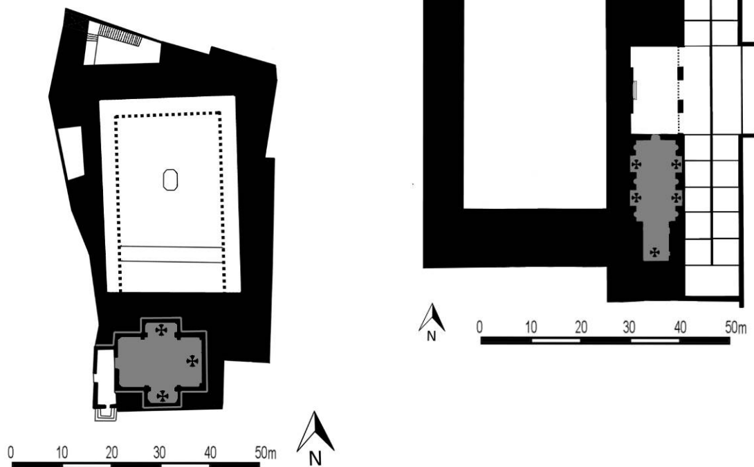
5. Plans restitués des monastères des annonciades célestes de Gênes II (à gauche) et de Sanremo (à droite). Croquis de l'autrice.
